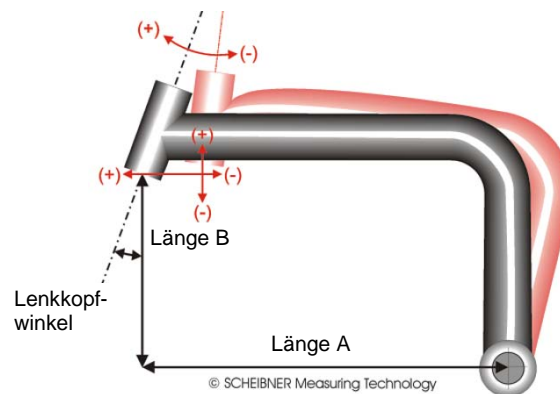
Ansicht: seitwärts
